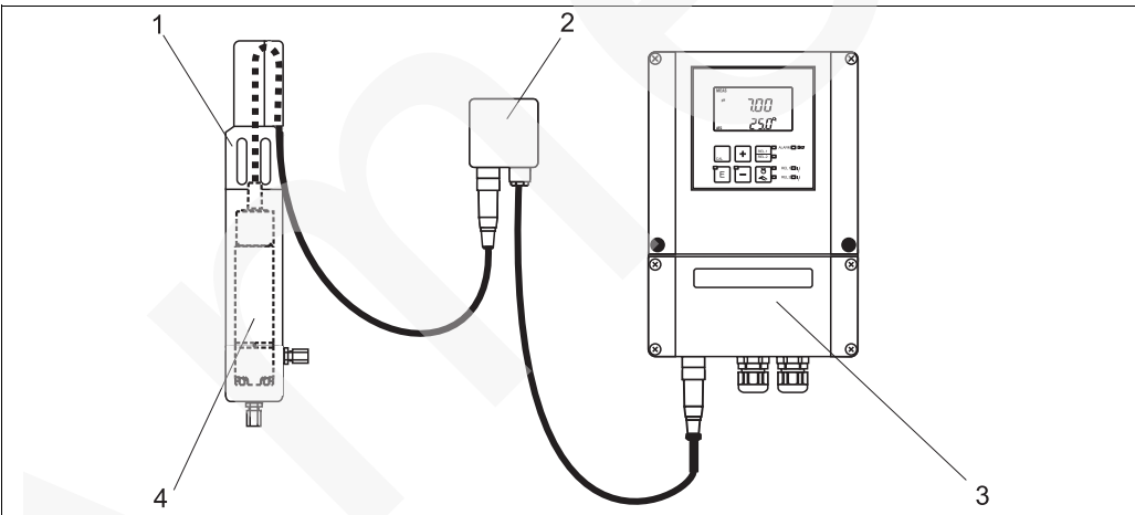
测量系统的结构示意图 1 流通式安装支架 2 VS 接线盒 (可选) 3 Liquisys M OOM253 变送器 4 溶解氧传感器
