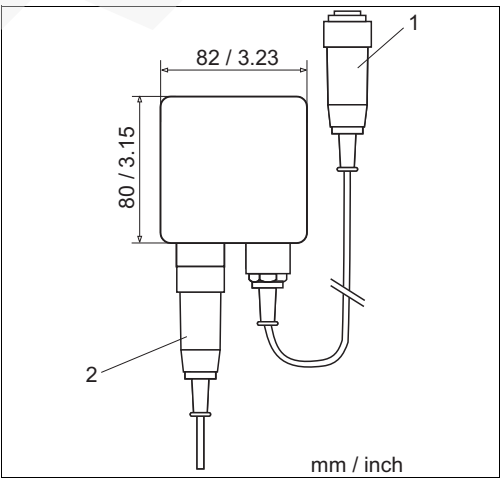
VS 接线盒与现场型设备的连接示意图
