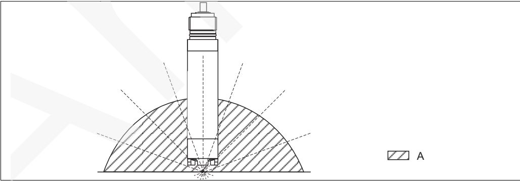
安装角度的示意图 A 允许安装角度范围: 0 ... 180 °
