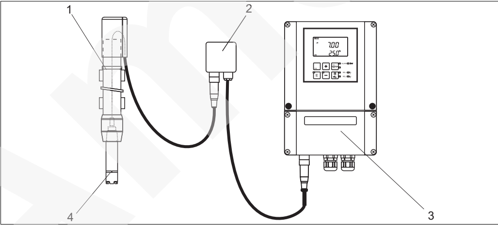
测量系统的结构示意图 1 浸入式安装支架 2 VS 接线盒 (可选) 3 Liquisys M OOM253 变送器 4 溶解氧传感器
